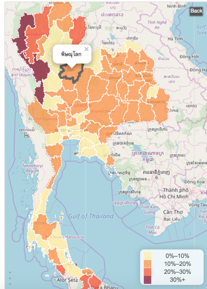
แผนที่แสดงร้อยละจำนวนนักเรียนยากจนพิเศษจากนักเรียนทั้งหมดรายจังหวัด
