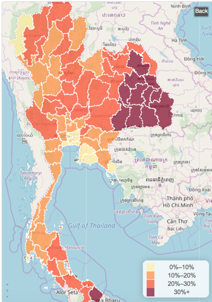
แผนที่แสดงร้อยละจำนวนนักเรียนยากจนจากนักเรียนทั้งหมดรายจังหวัด
